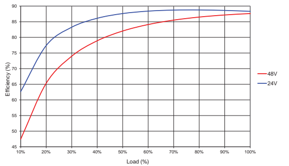
NCS12S4815C
