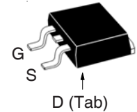
TO-263AA (IXFA)
